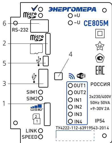
Рисунок 3 – Передняя панель УСПД с трехфазным подключением к сети переменного тока
