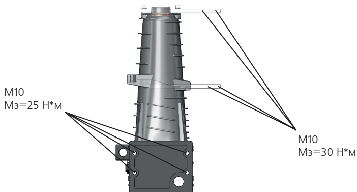
Рисунок 11 — Точки крепления коммутационного модуля
