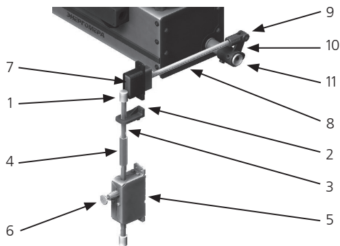
Рисунок 7 — Блокировочное устройство. 1 — упор; 2 — кронштейн; 3 — тяга; 4 — муфта; 5 — блокиратор; 6 — фиксатор; 7 — кнопка ручного отключения; 8- шпилька М10; 9 — вилка; 10 — рычаг; 11 — втулка.
