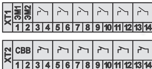
Рисунок 4 — Обозначение разъемов вторичной коммутации коммутационного модуля
