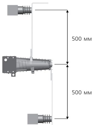
Рисунок 13 — Максимально допустимая длина пролетов шин
